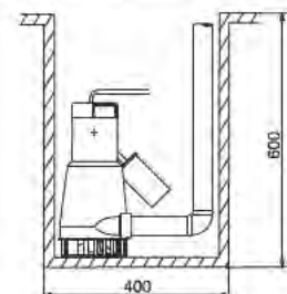
FEKA 300 - FEKA 600
