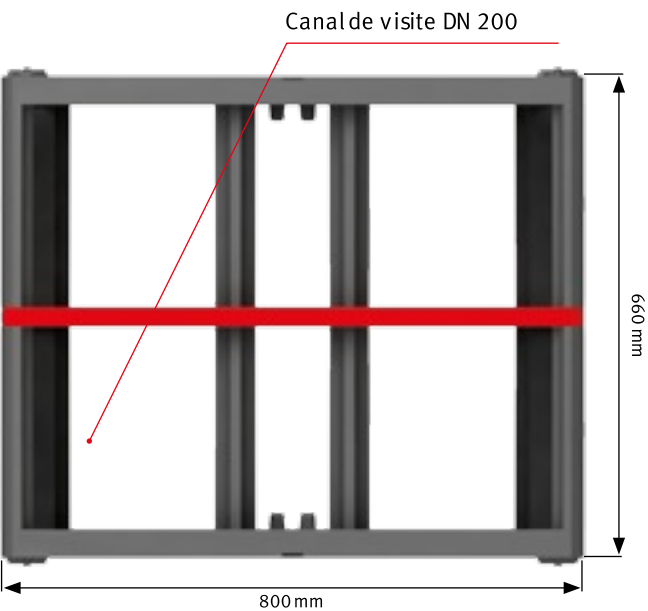
EcoBloc inspectable 420 : vue de face
